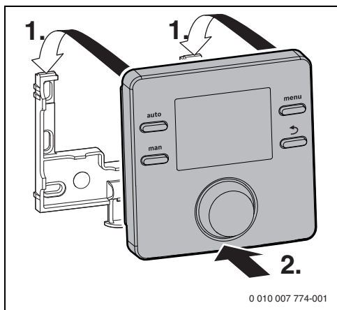
SI.5 Vpenjanje regulatorja
