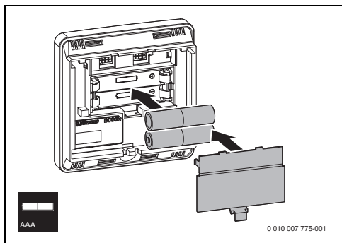
SI.4 Vstavite baterije
