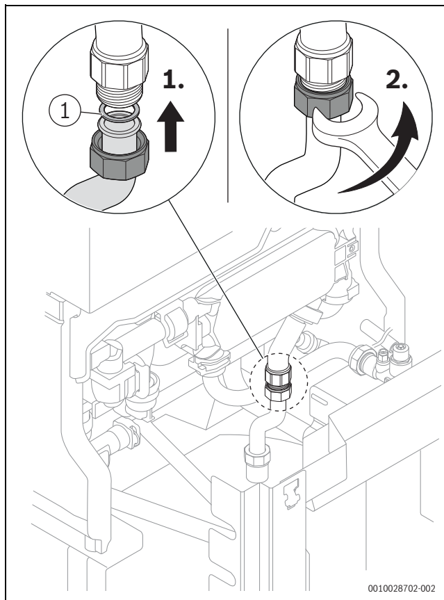
Sl.63 Cev za toplo vodo bojerskega kroga priključite na boiler.
