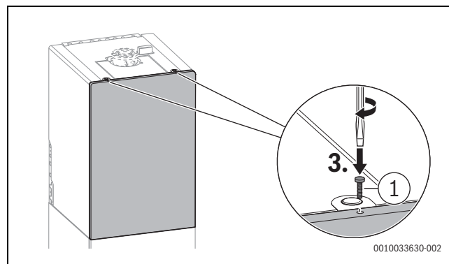
Sl.94 Pritrjevanje prednjega dela obloge naprave z vijakom iz obsega dobave
