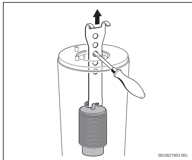
Sl.126 Odstranjevanje spodnjih izpodravnih elementov
