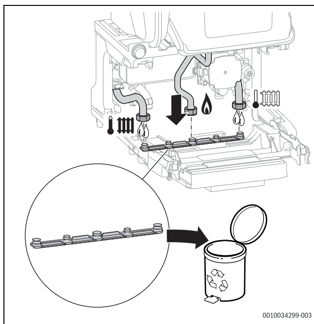
Sl.56 Odstranite pokrivno letev iz naprave
