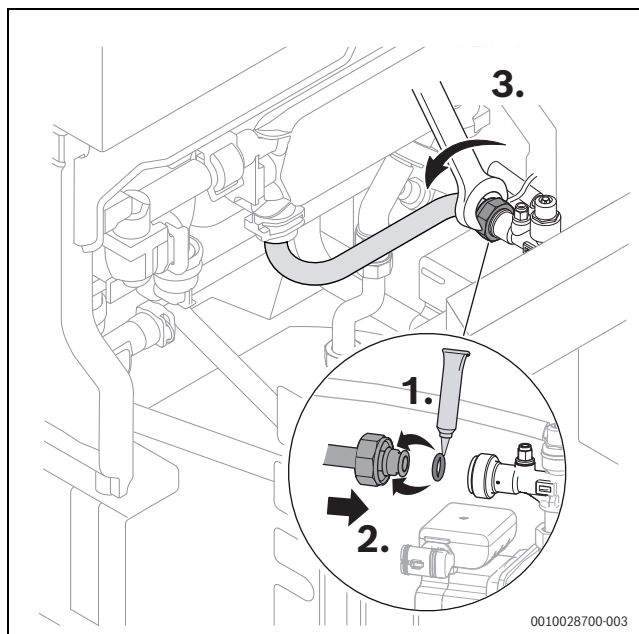
Sl.62 Priključite cev za hladno vodo bojerskega kroga.
