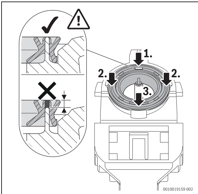
Sl. 150 Pritisk tesnila navzdol
