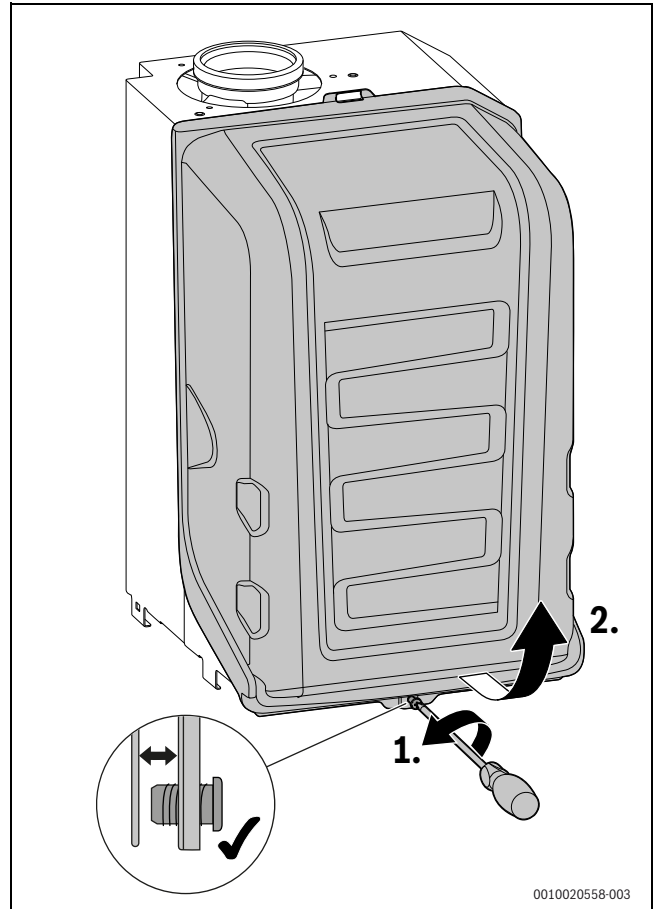
Sl. 104 Odstranitev pokrova gorilnika
