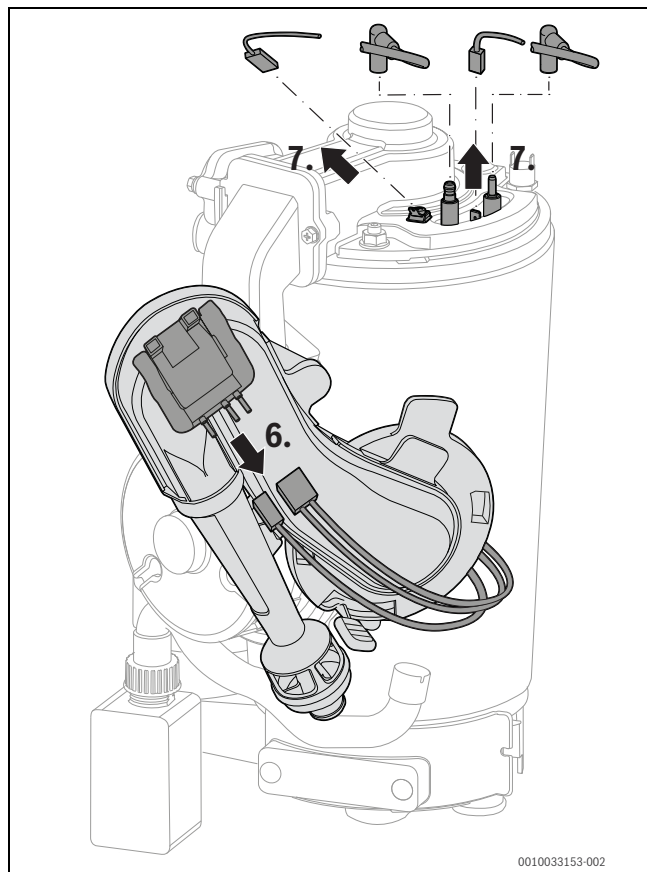
Sl.120 Snemanje kabla
