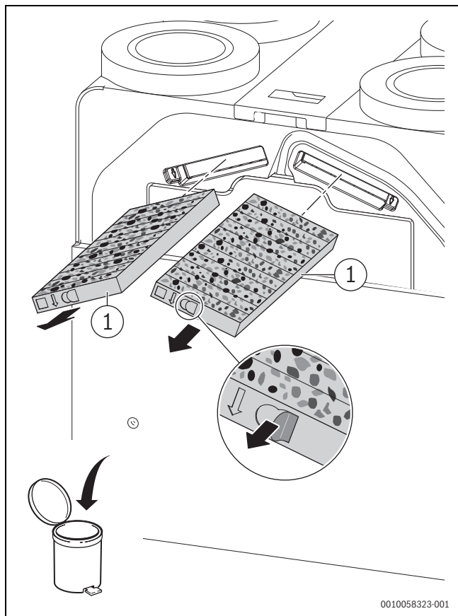
Sl.8 Odstranjevanje filtrov
