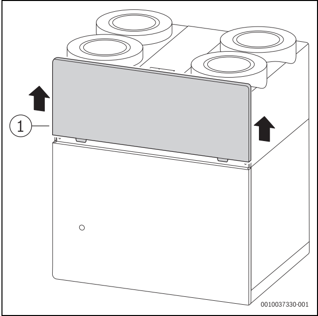
Sl. 6 Odstranjevanje (kovinskega) pokrova filtrov
