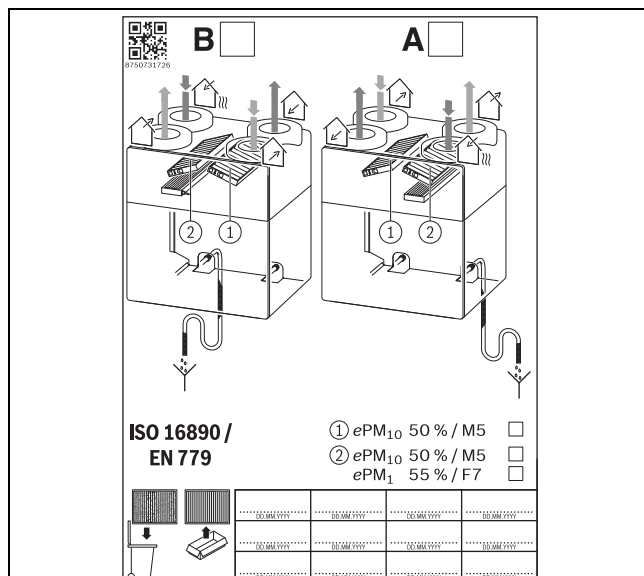
Sl.11 Nalepka za menjavo filtrov
