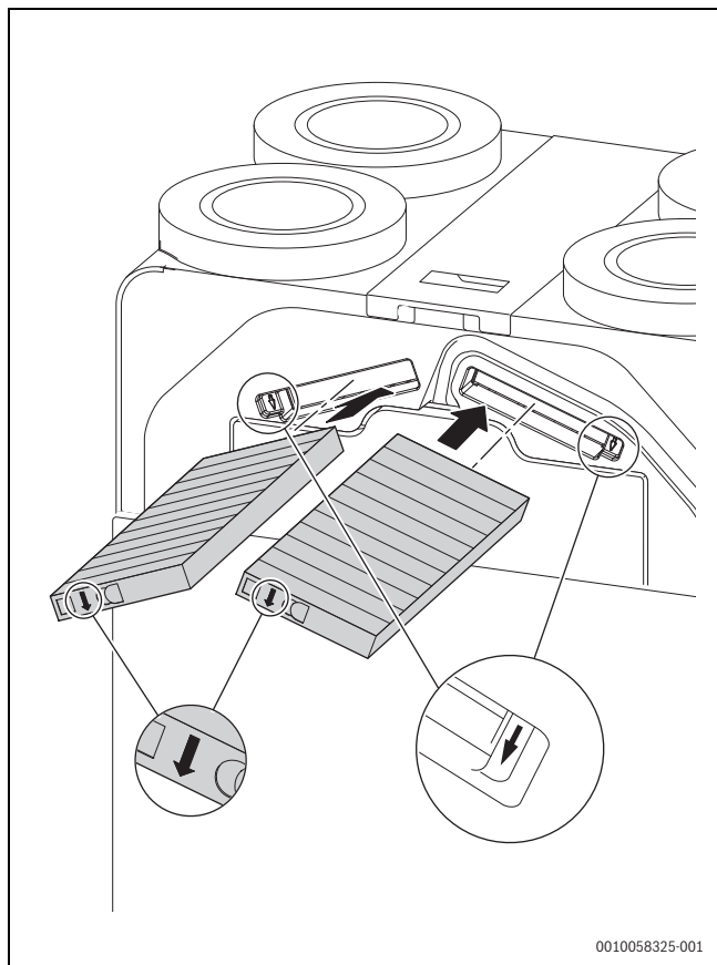
Sl.9 Vstavljanje filtrov
