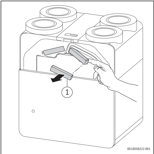
Sl. 7 Odstranjevanje filtrov
