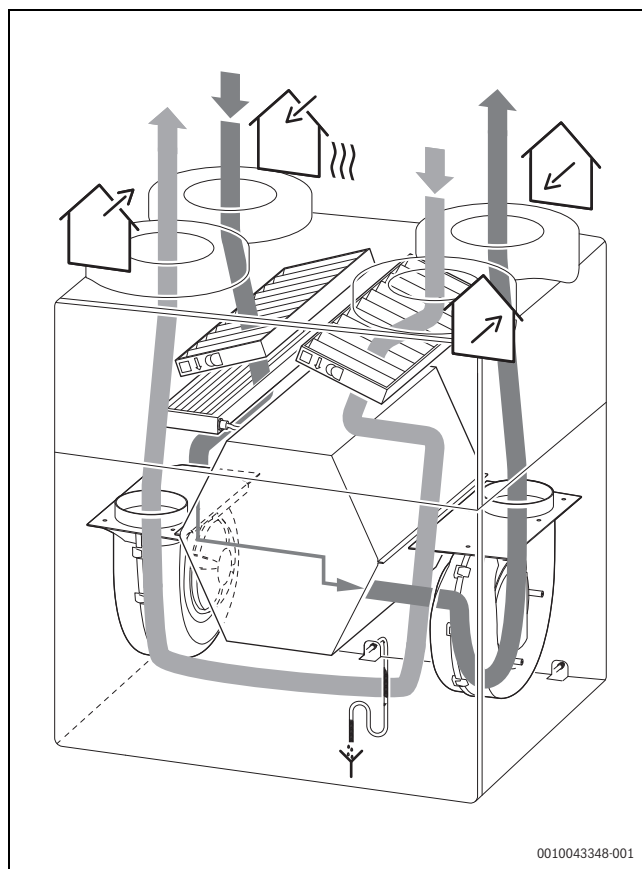
Sl.4 Primer vodenja zraka pri obratovanju z obvodom pri različici B
