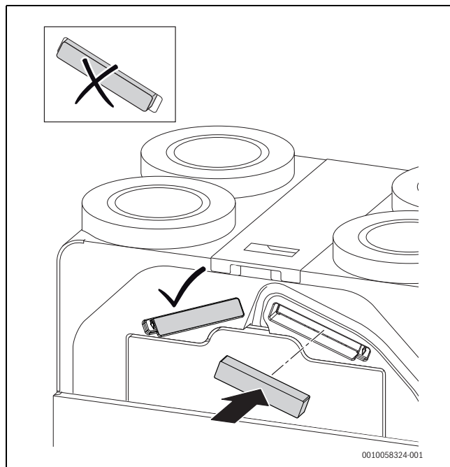
Sl.10 Montaža pokrova filtrov
