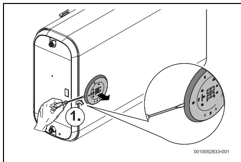
Rys. 11 Odłączanie wyświetlacza
