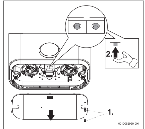
Fig. 15 Termostat de siguranță
