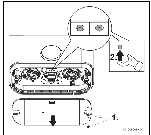
Σχ. 15 Θερμοστάτης ασφαλείας
