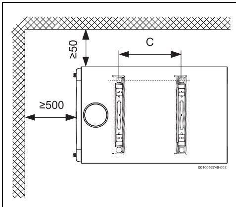
Σχ. 3 Διαστάσεις σε mm (επιτοίχια, οριζόντια εγκατάσταση)
