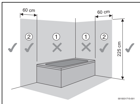
Rys. 6 Strefa ochronna
