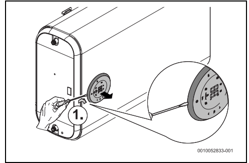
Fig. 11 Scoaterea afișajului
