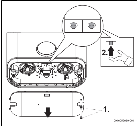
sl. 15 Sigurnosni termostati
