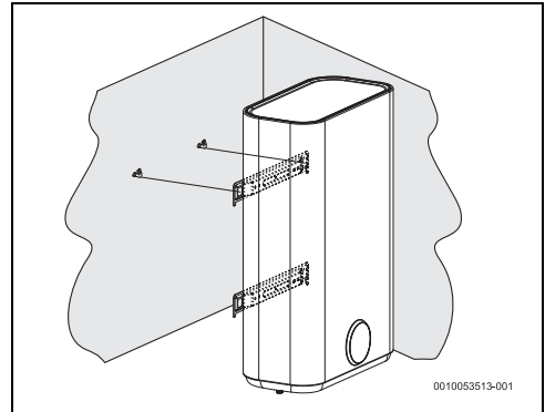
8. ábra Független telepítés (falra szerelés)
