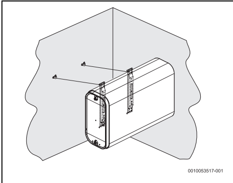
fig. 10 Instalim horizontal (montim në mur)
